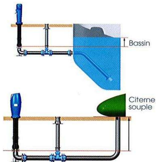
Principe d'implantation d'un poteau d'aspiration
